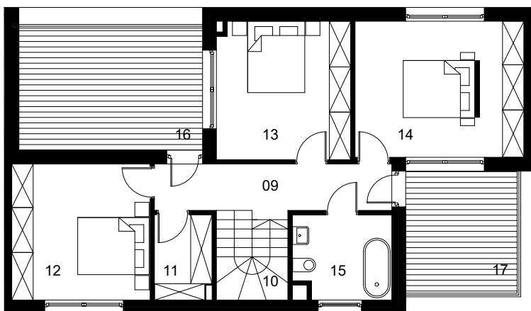
RZUT PIĘTRA
