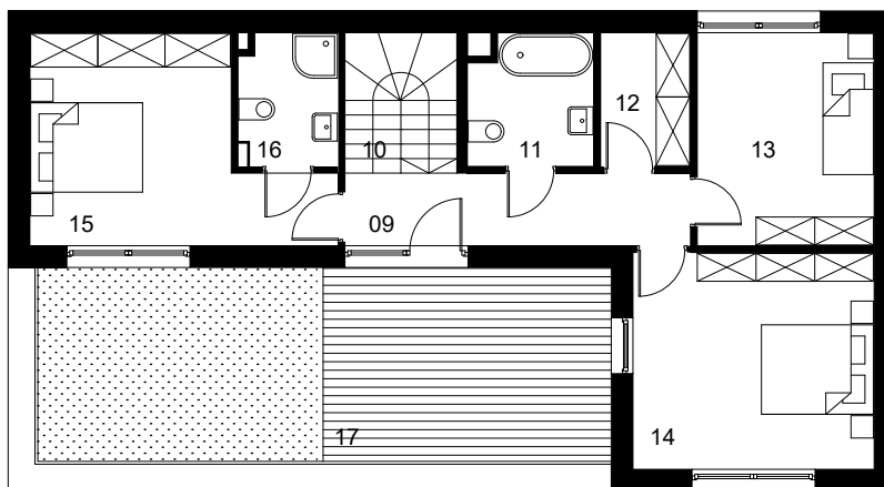
RZUT PIĘTRA
