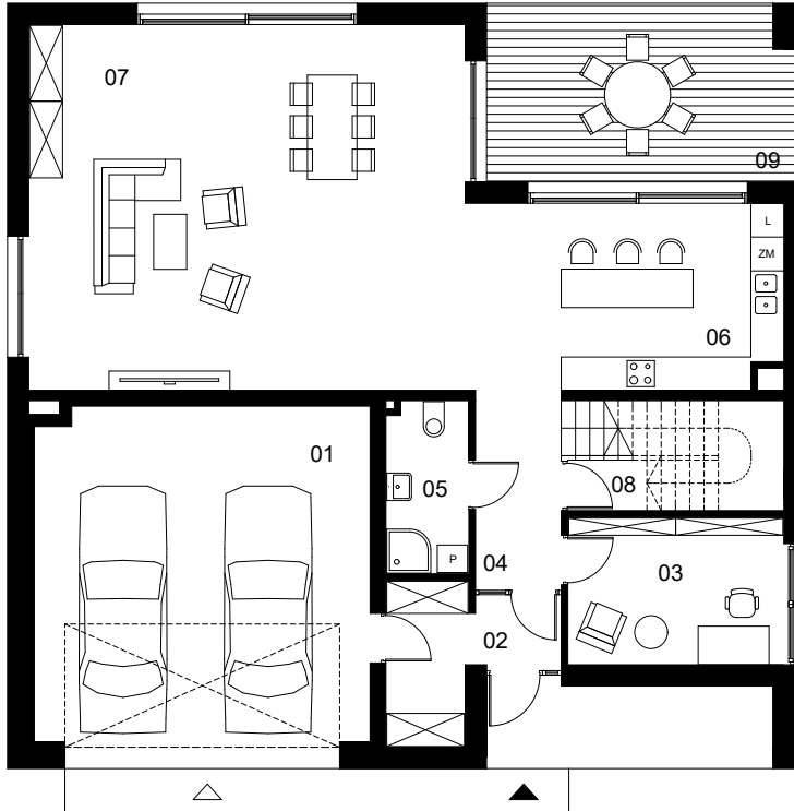
RZUT PARTERU
