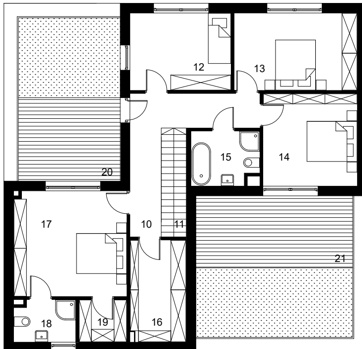
RZUT PIĘTRA
